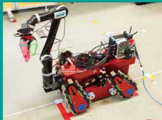
「World Robot Summit 2020」に向けて会津大学が地元企業と協同開発した災害対応ロボット「スパイダー2020」
